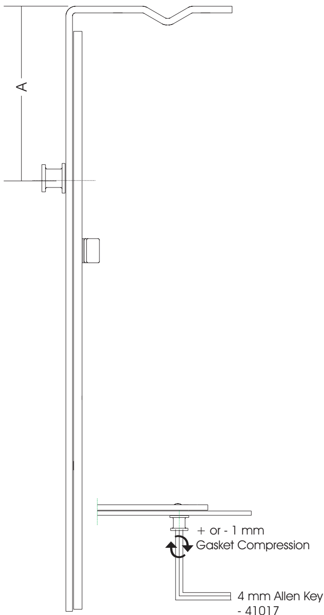
MACO Espagnolette Fittings
