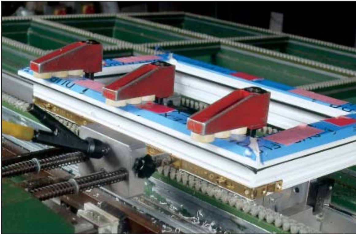
„Click-Fix“ - Eurogroove clips
